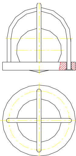
球笼组合
