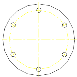
隔膜
