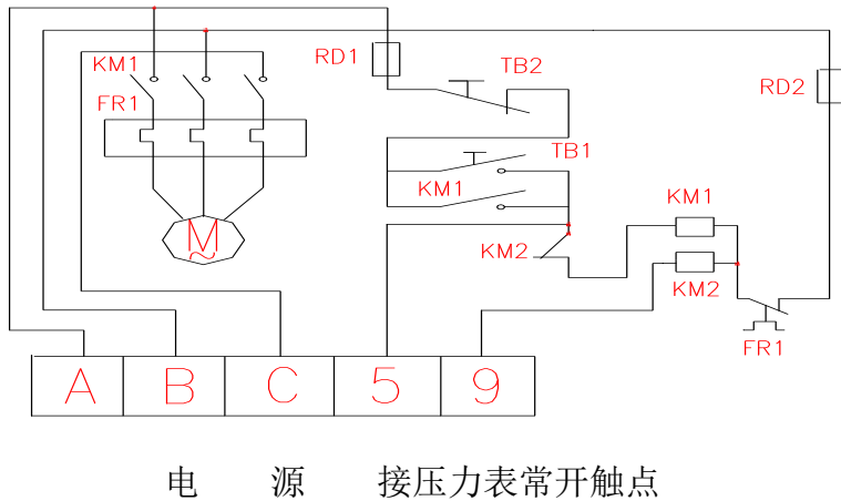
图三 电气控制原理图
