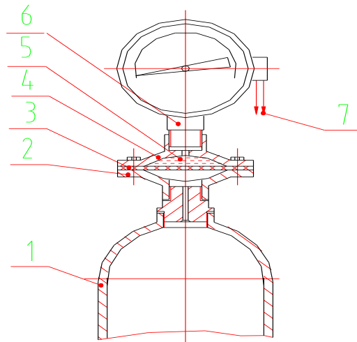
图二 压力安全装置
